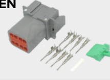
RS931008-2 PINNARUNKOSARJA 8-NAPAINEN
