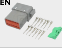
RS931012-2 PINNARUNKOSARJA 12-NAPAINEN
